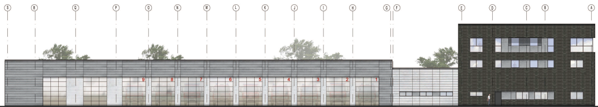
Ansicht Westen
