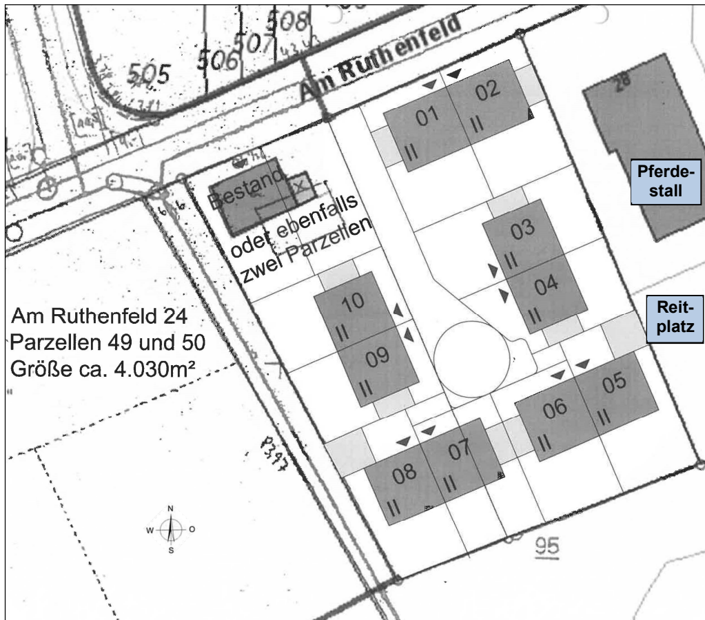
Abb. 2: Entwurf des Bebauungskonzeptes (Ausschnitt) /9/
