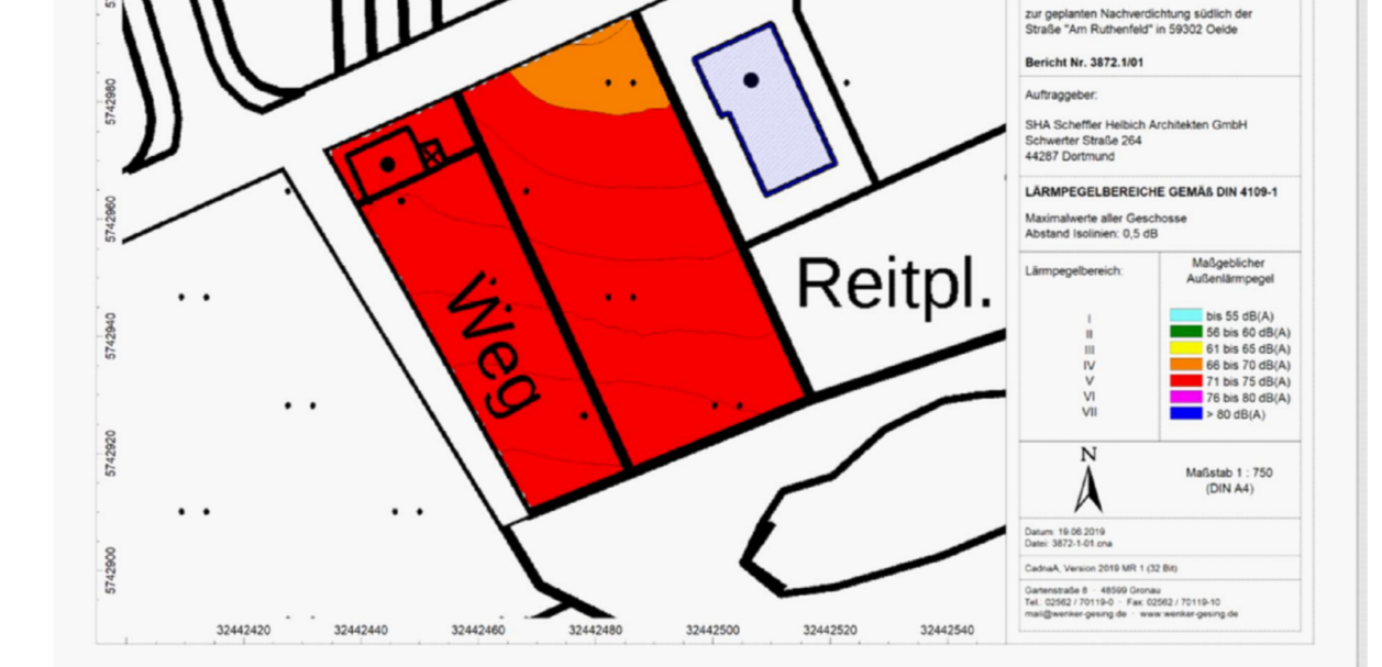
Lärmkarte Verkehr, Lärmpegelbereiche aller Geschosse bei freier Schallausbreitung, Wenker & Gesing 2019
