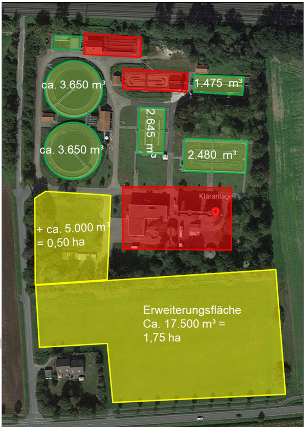
Abbildung 18: Grafische Lagaplandarstellung der Bestandsbewertung Verfahrenstechnik im Ausbauzustand 70.000 EW
