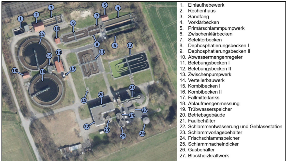
Abbildung 3: Aufbau der Kläranlage Oelde mit nummerierten Anlagenenteilen
