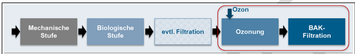
Abbildung 35: Einfaches Grundfließschema der Abwasserreinigung mit Ozonung und BAK-Filtration
