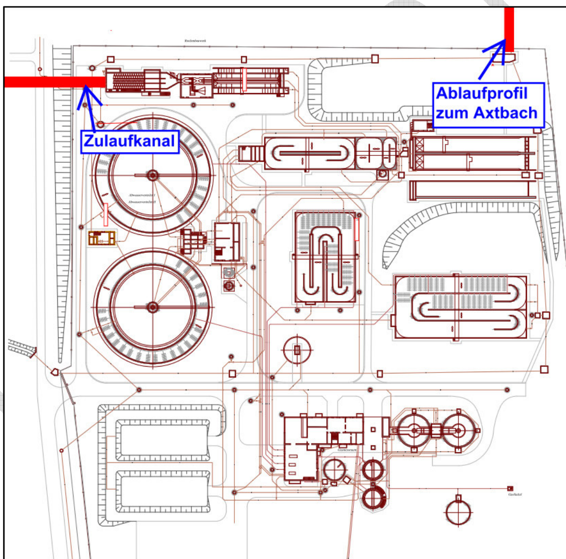
Abbildung 19: Lageplan der KA Oelde mit Kennzeichnung des Zu- und Ablaufkanals
