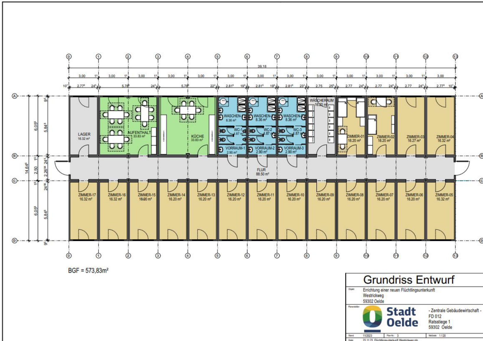
Westrickweg – beispielhafter Grundriss
