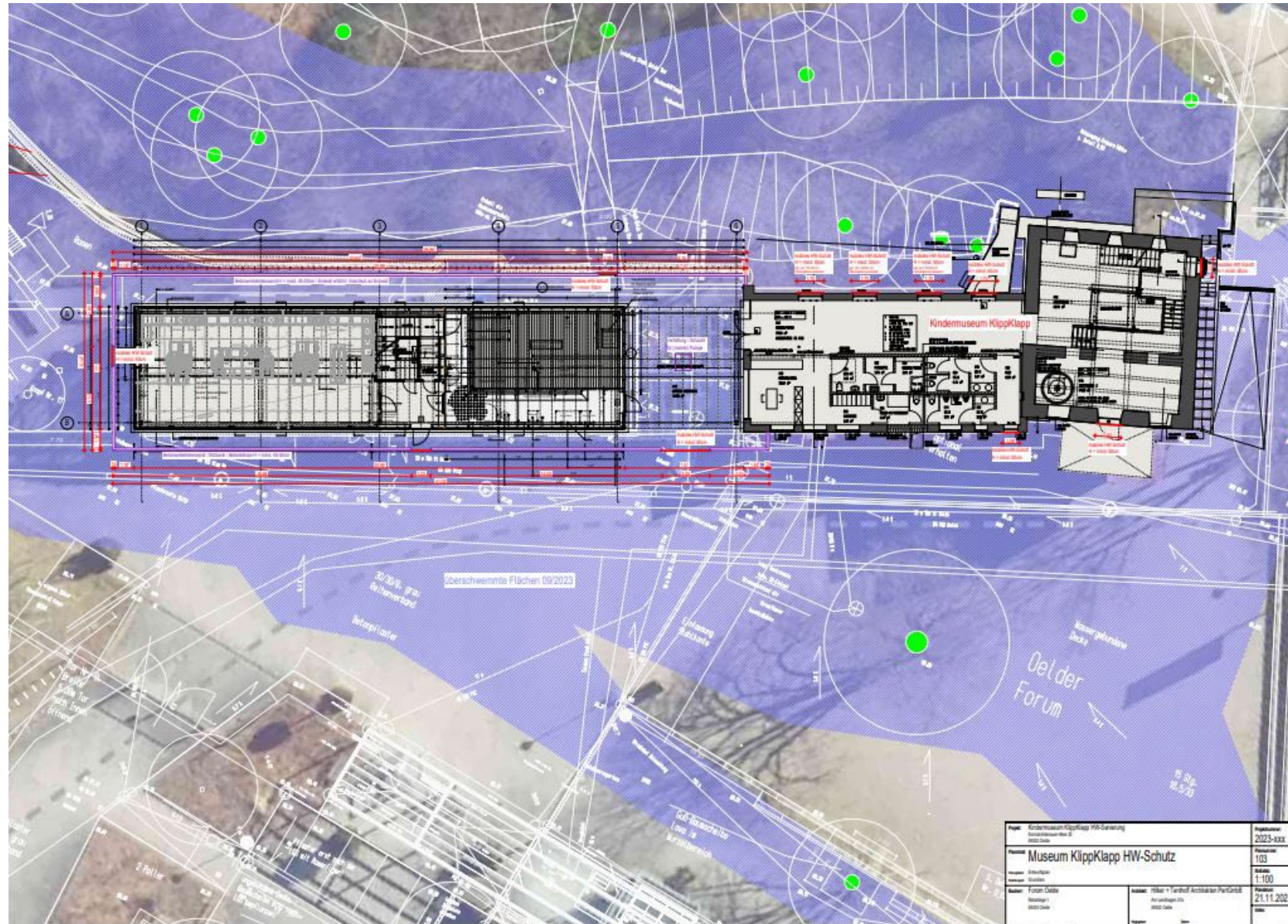
Bauliche Maßnahmen Hochwasserschutz Kindermuseum KlippKlapp
