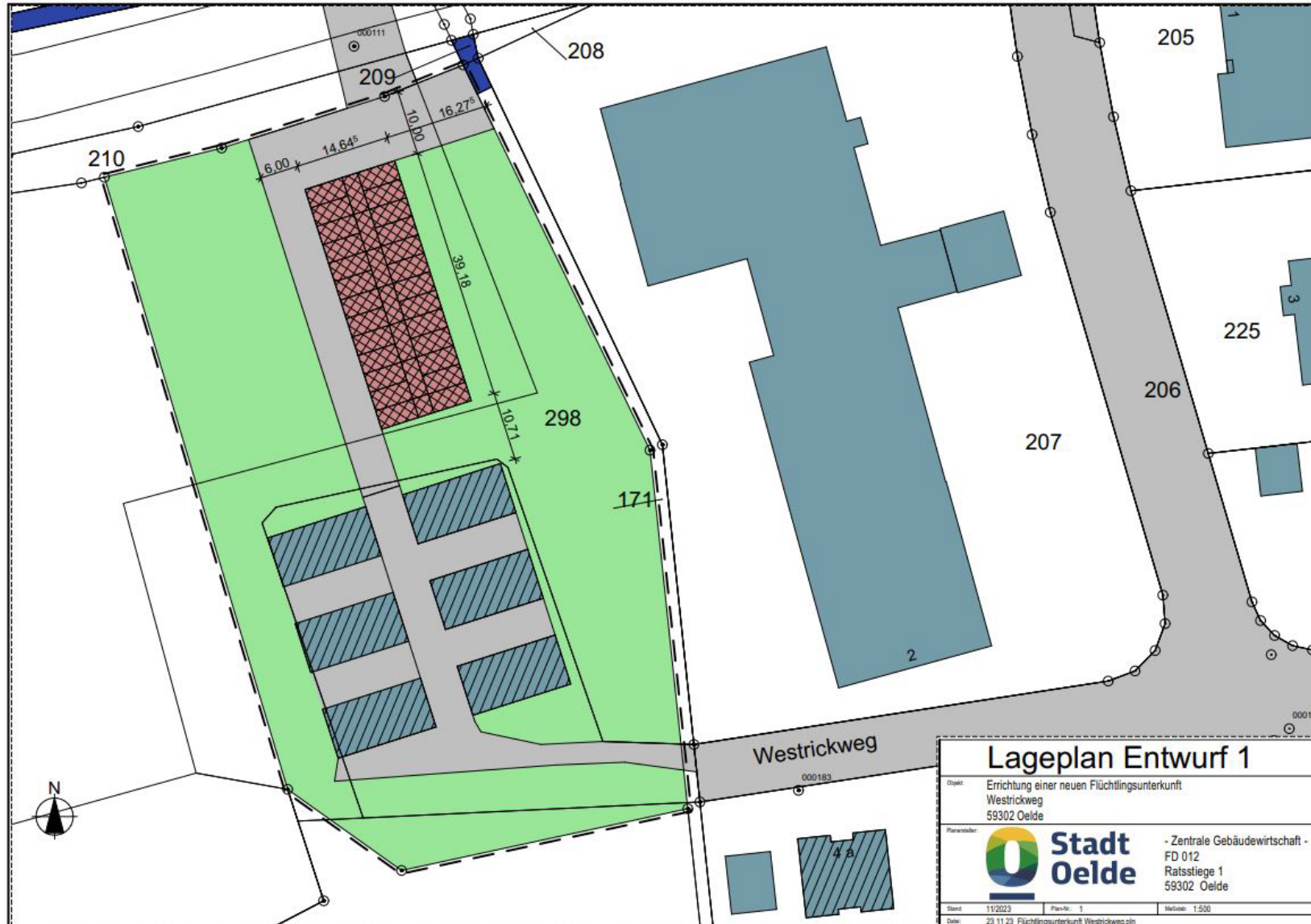
Lageplan Westrickweg - zweigeschossig
